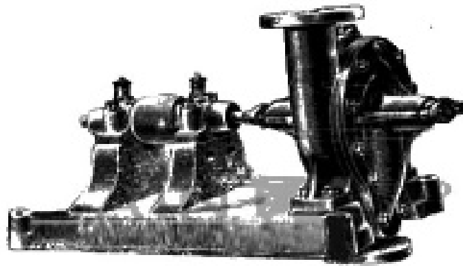
طلمبا لسحب الماء من الآبار والآبار ورقيها إلى محل عالي لسقي الأراضي
